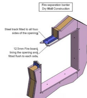
Fig. 3: Drywall Construction
